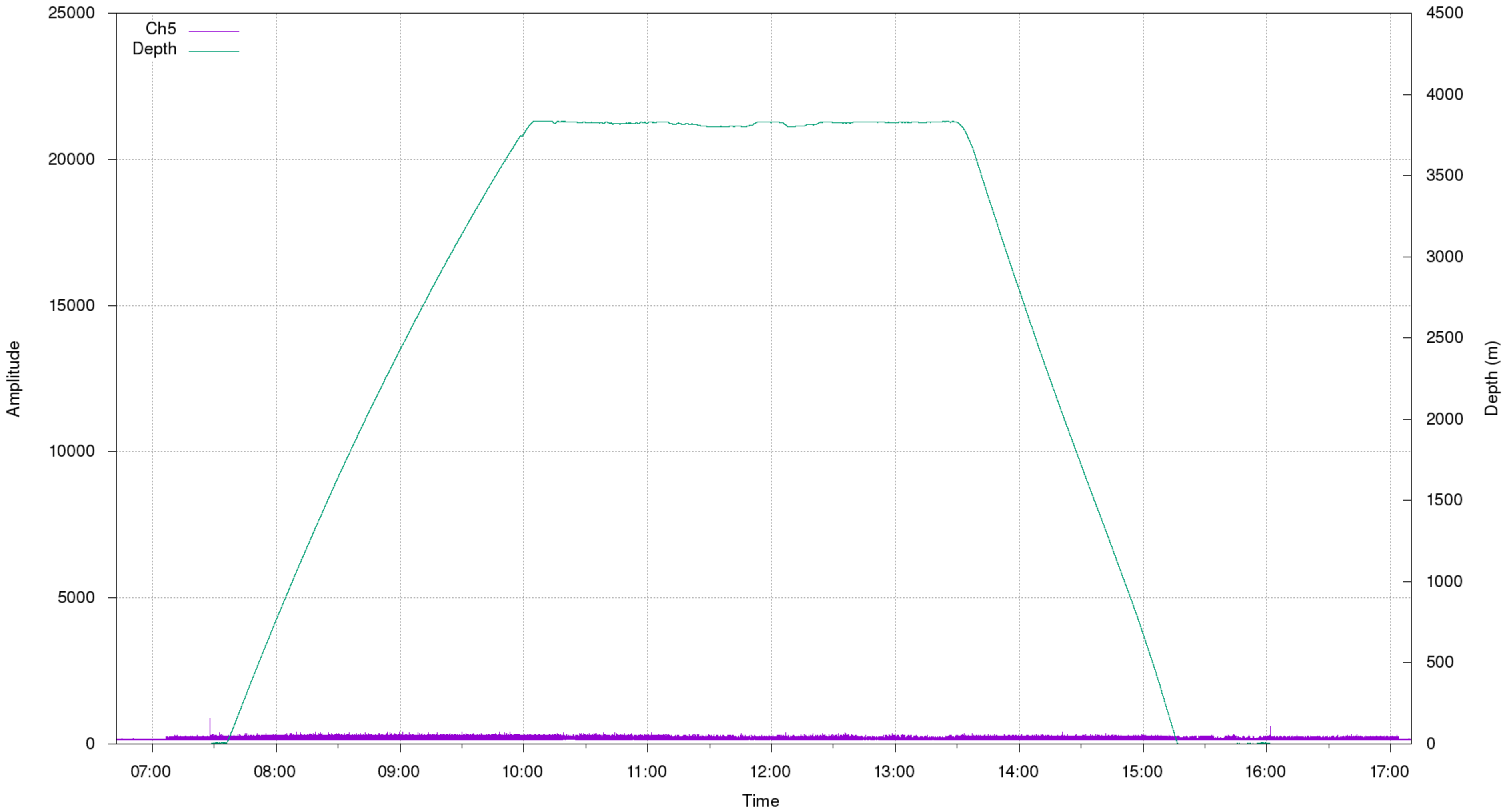
AE Max Amplitude 071522021236 | Ch5
