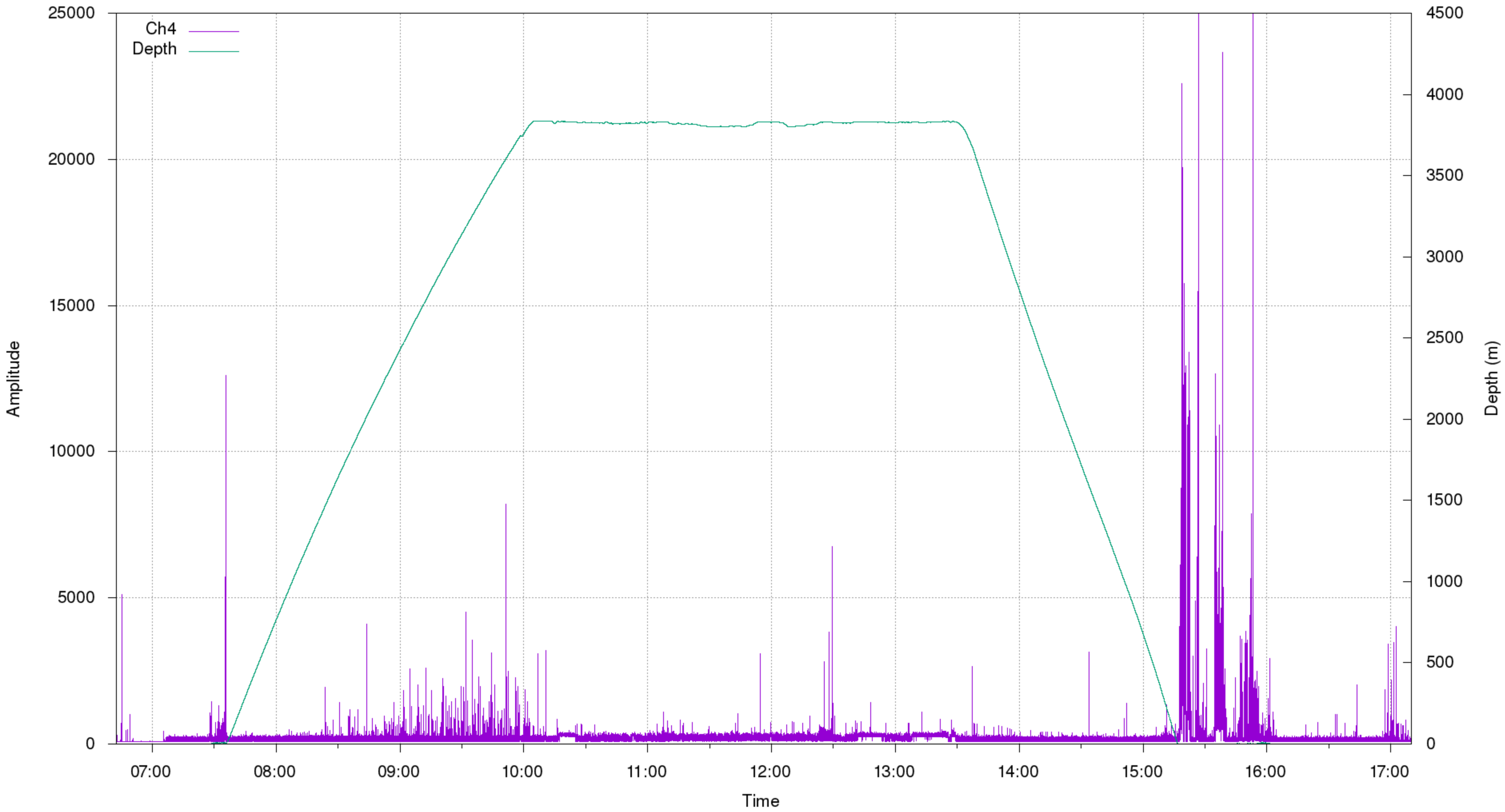
AE Max Amplitude 071522021236 | Ch4
