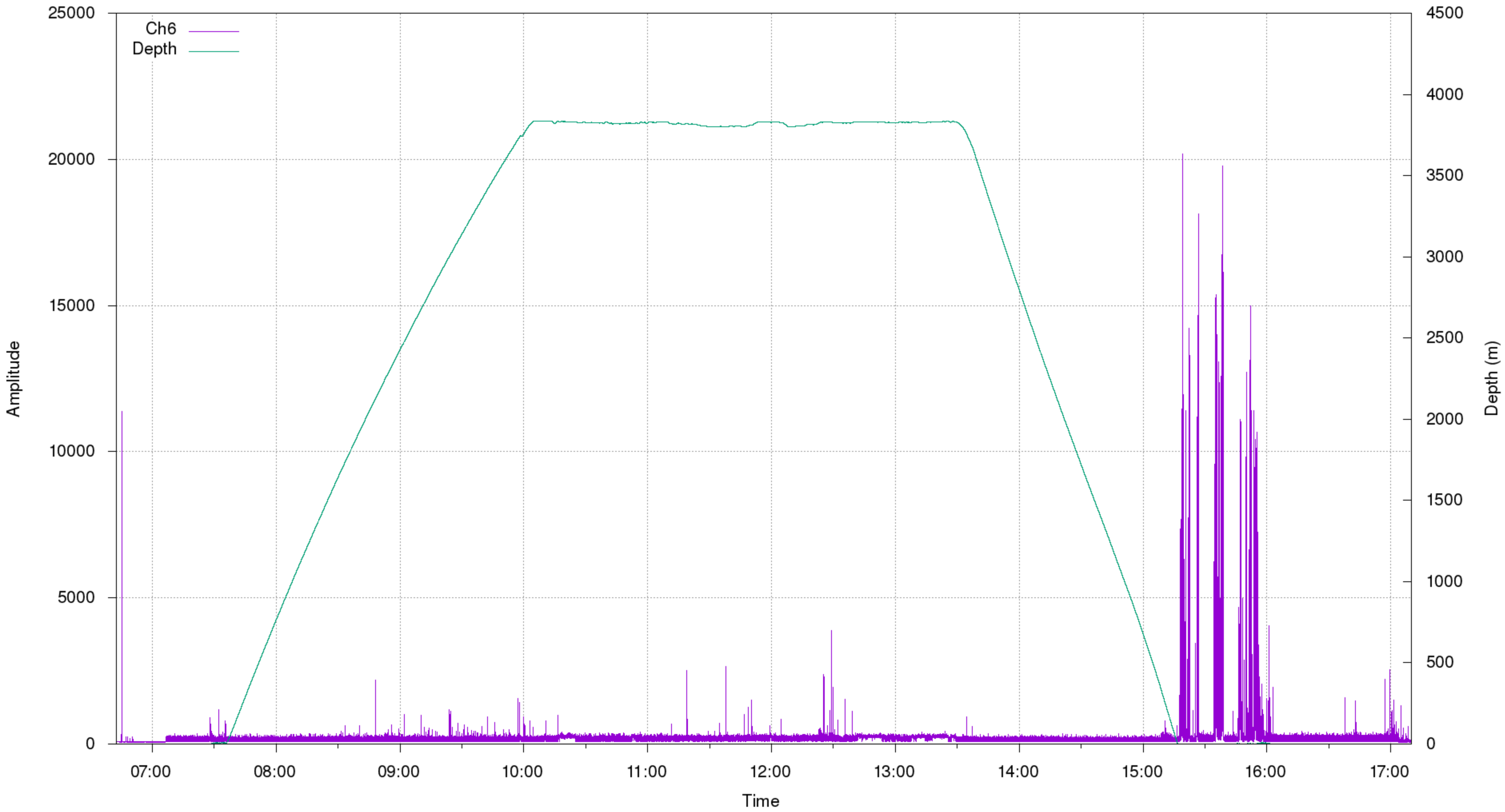
AE Max Amplitude 071522021236 | Ch6
