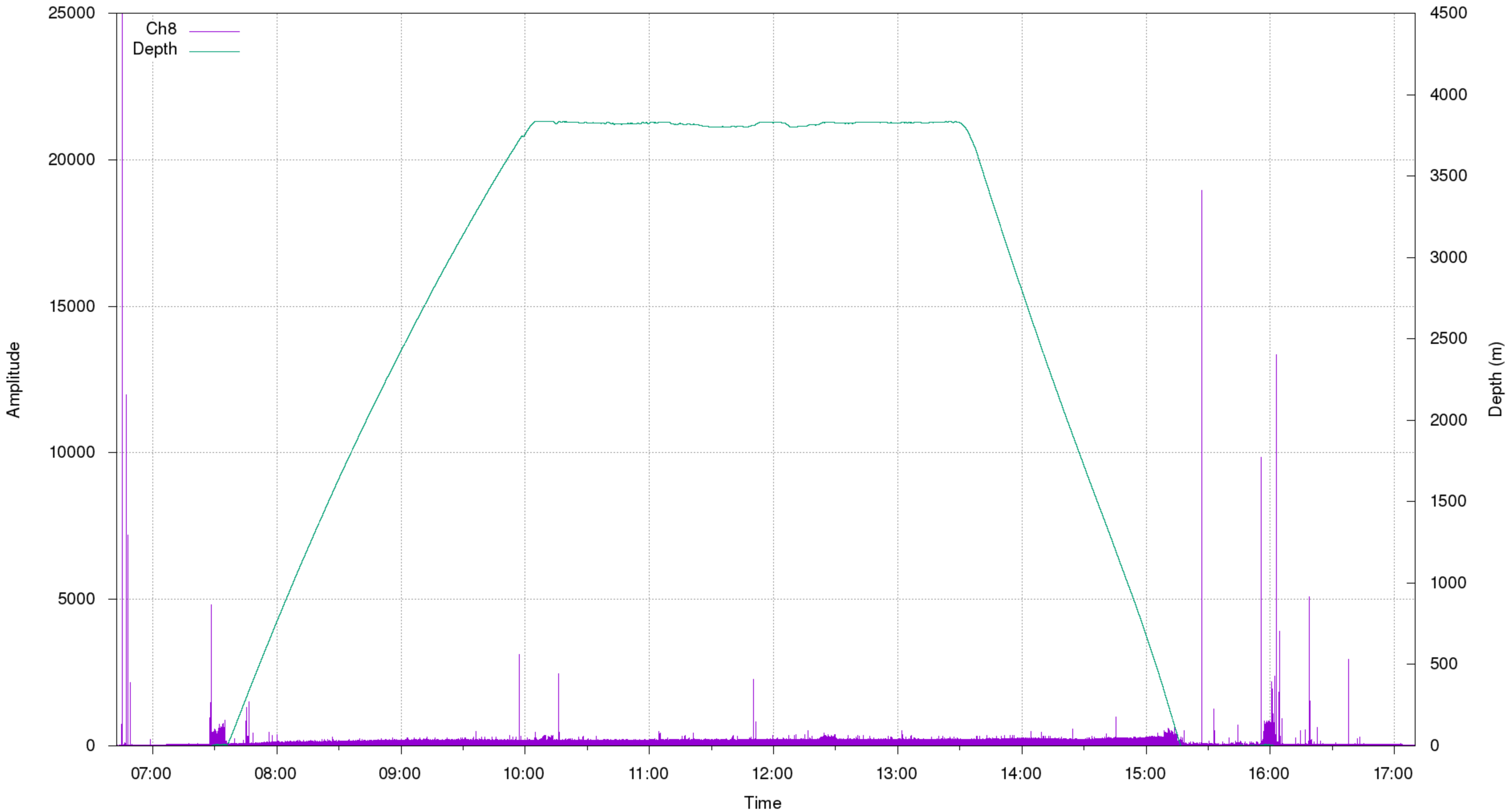
AE Max Amplitude 071522021236 | Ch8
