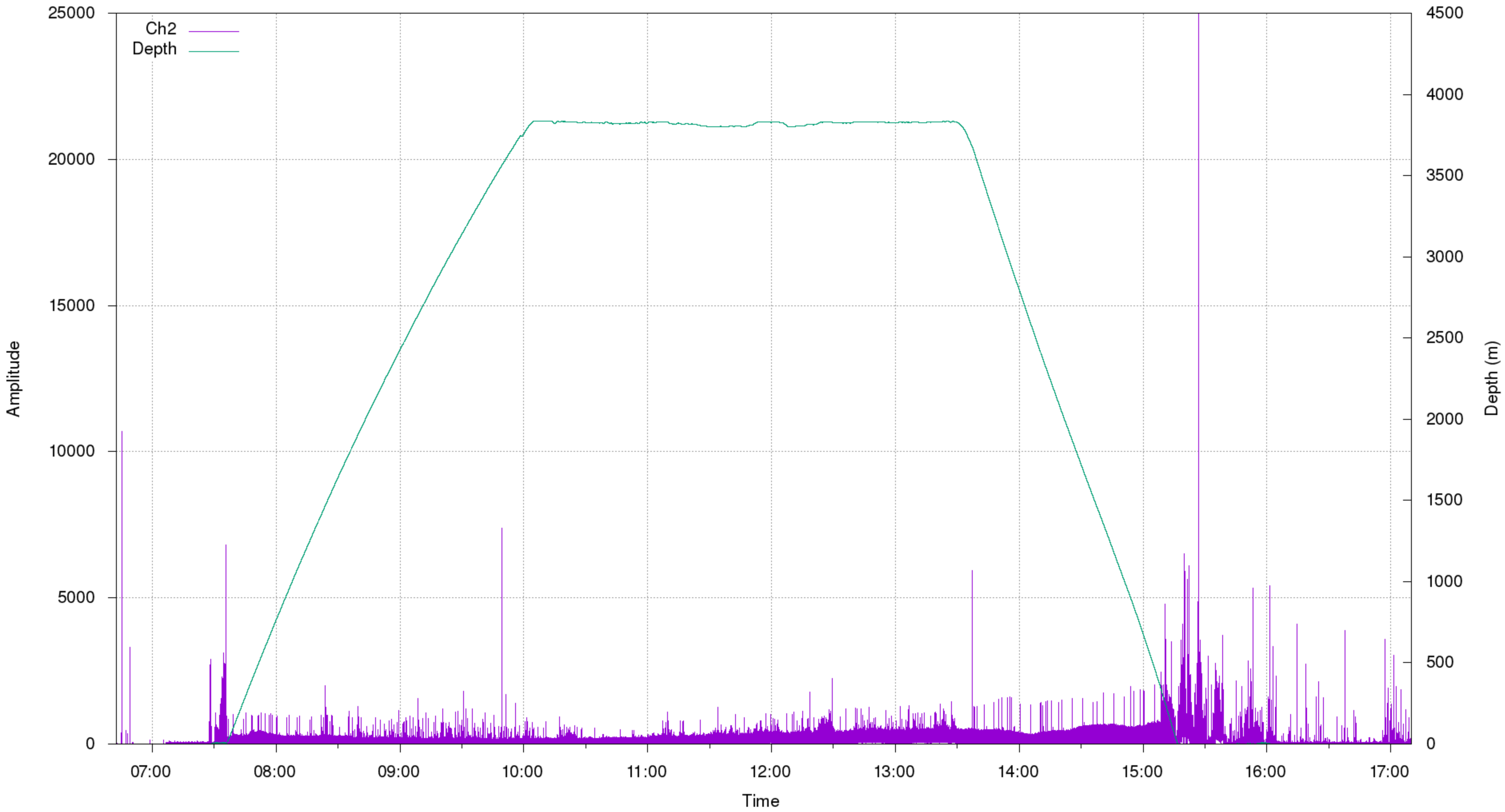
AE Max Amplitude 071522021236 | Ch2
