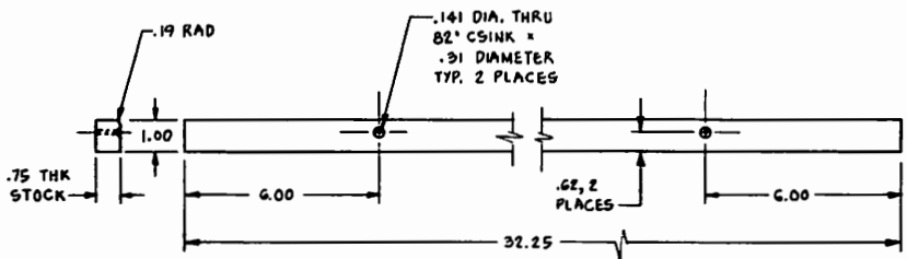
(-42) CONTOUR EDGING, STRAIGHT
