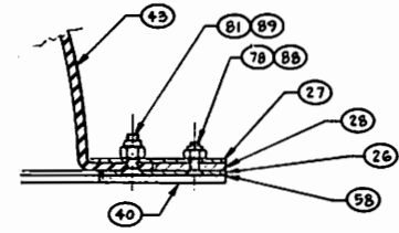
SECTION 13-13 SCALE: 1/1
