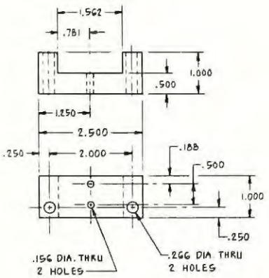
(-33) FEEDER GUIDE BLOCK SCALE: \frac{1}{1}
