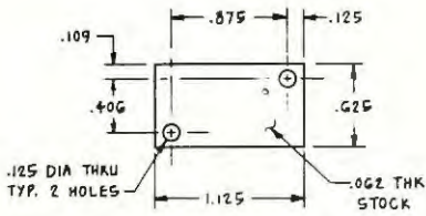
(-35) LIMIT SWITCH SPACER SCALE: \frac{2}{1}
