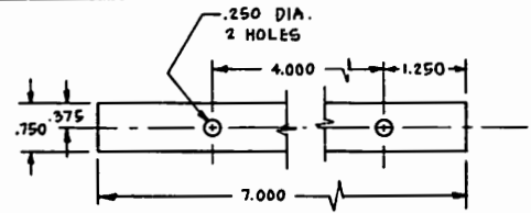
(-7) FASTENER, FILE, ST&D
