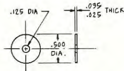
(-34) BEARING WASHER SCALE: \frac{2}{1}
