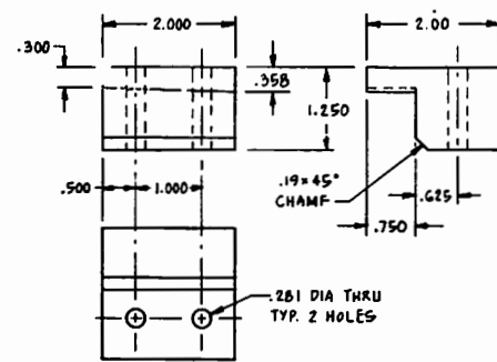
(-31) MOUNT, FWD - STBD SCALE: \frac{1}{1}
