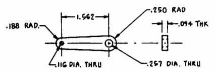
(-20) MOTOR ARM SCALE: \frac{1}{4}
