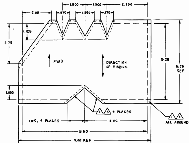
(-2) HARNESS SCALE: \frac{1}{1}
